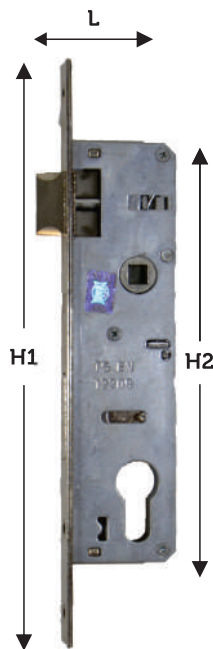
Broască KALE CU LIMBĂ
