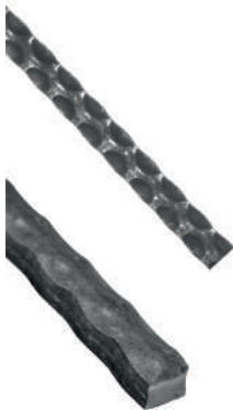
Oțel pătrat amp. pe cant L: 6000 mm
